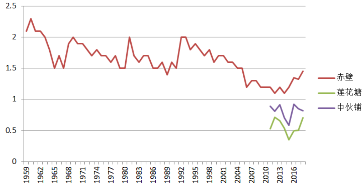
图 3.2-3 (d) 建站至 2018 年平均风速年际变化
