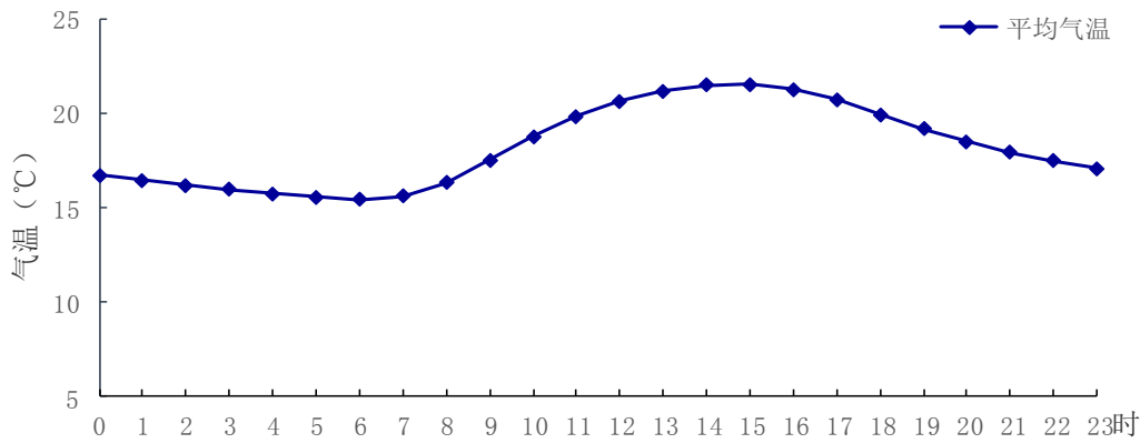
图 4.2-5 赤壁气象站累年（2009-2018 年）平均气温日变化
