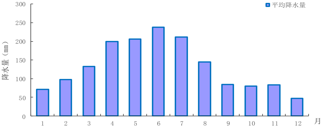
图 4.3-2 赤壁气象站累年（1989-2018 年）降水量年变化
