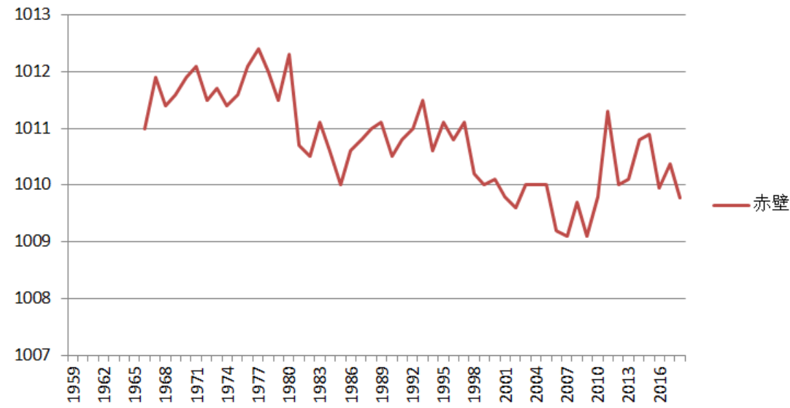
图 3.2-3 (b) 建站至 2018 年平均气压年际变化
