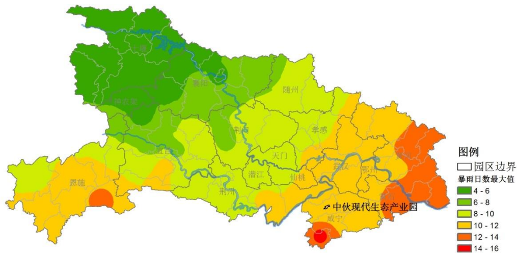
图 5.1-8 1961-2018 年湖北省年暴雨日数极大值分布图
