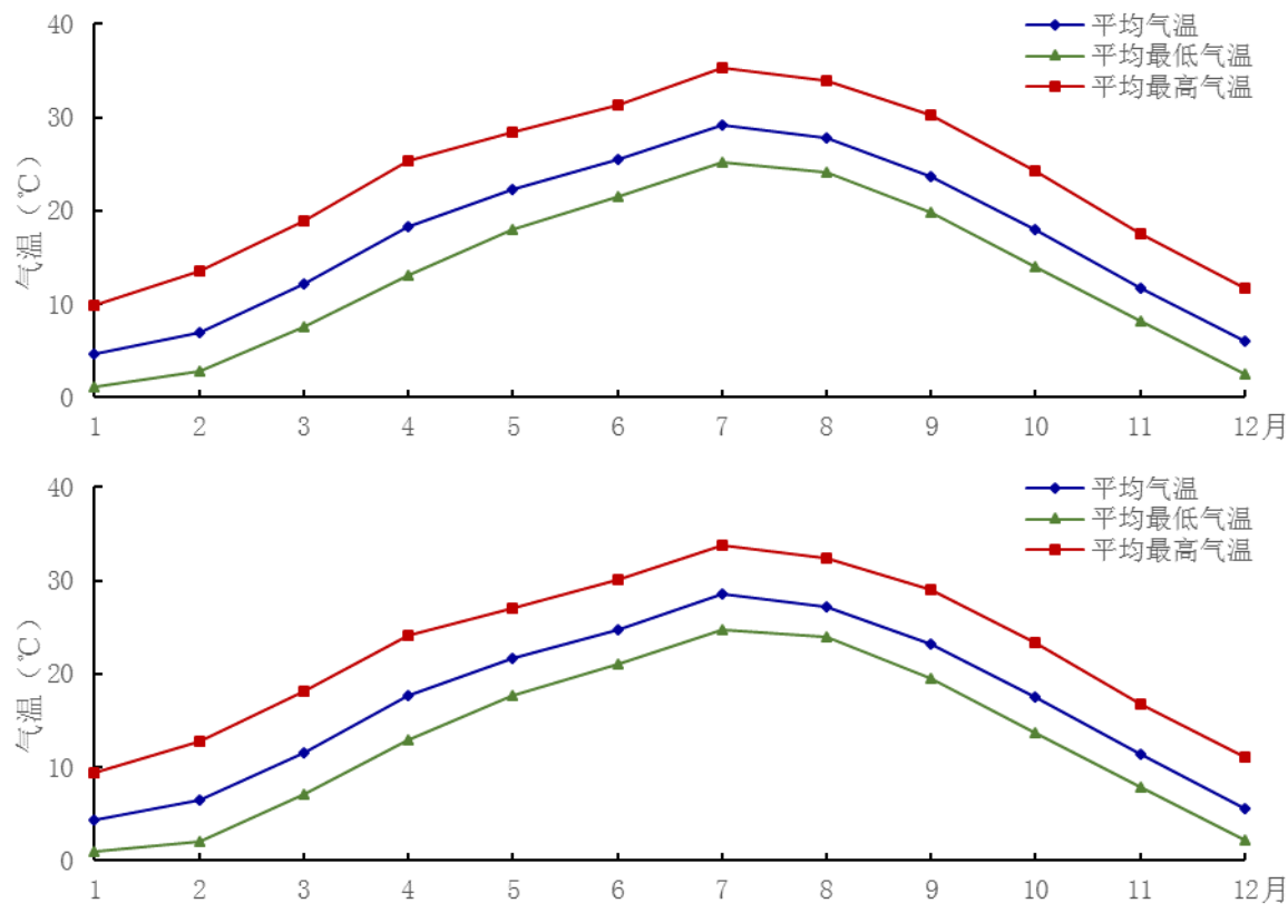
图 4.2-5 赤壁气象站、中伙铺、莲花塘区域站（2016-2018 年） 平均气温、平均最高、平均最低气温年变化
