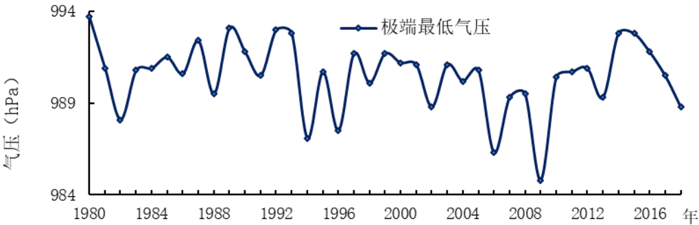
图 4.1-3 赤壁气象站 1980-2018 年极端最低气压年际变化
