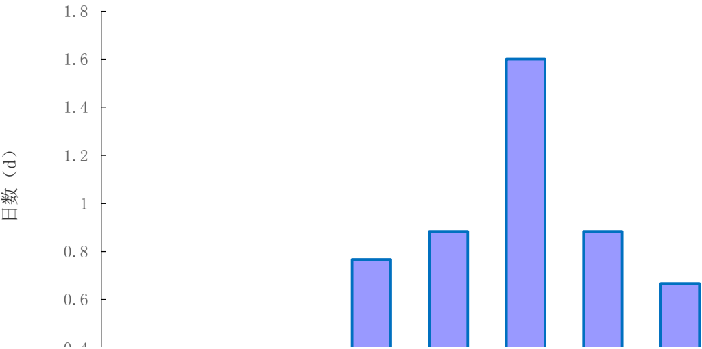
6.1-2 赤壁气象站累年（1959-2018 年）平均暴雨日数年变化
