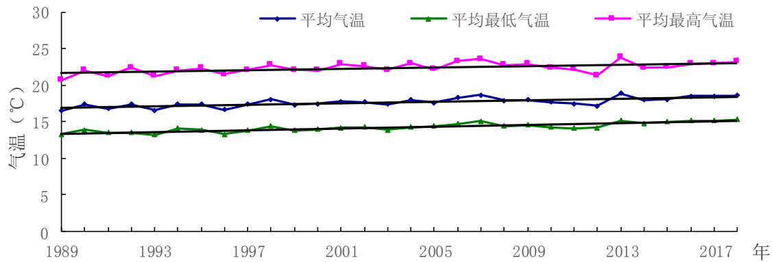
图 4.2-1 赤壁气象站 1989-2018 年平均气温、平均最高、平均最低气温年际变化
