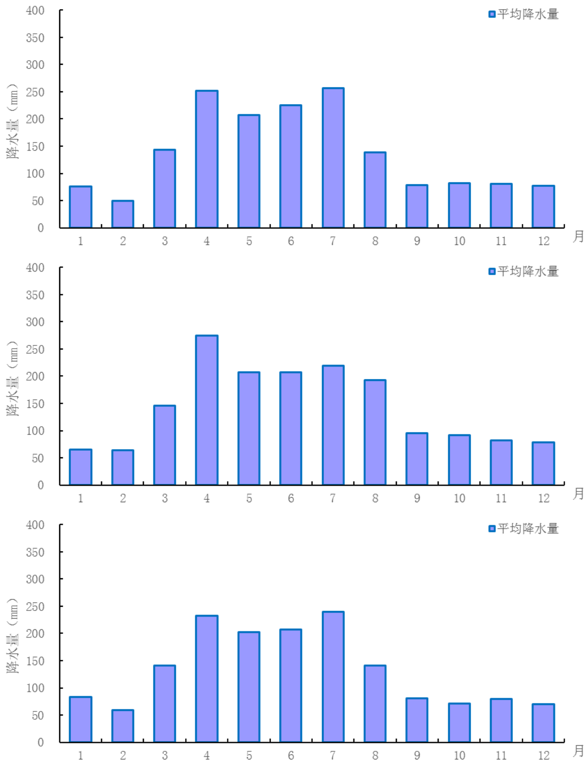
图 4.3-3 赤壁气象站、中伙铺、莲花塘区域站（2016-2018 年）降水量年变化
