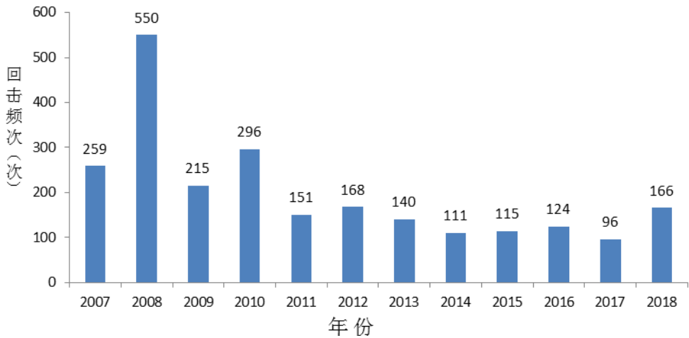
图 5.2-3 2007-2018 年赤壁中伙现代生态产业园及周边地闪回击年变化特征
