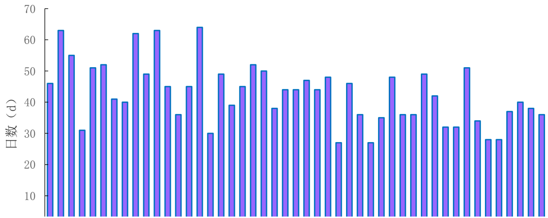
图 6.2-1 赤壁气象站 1959-2013 年雷暴日数年际变化
