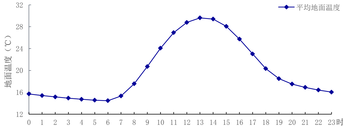
图 4.7-5 赤壁气象站累年（2009-2018 年）平均地面温度日变化
