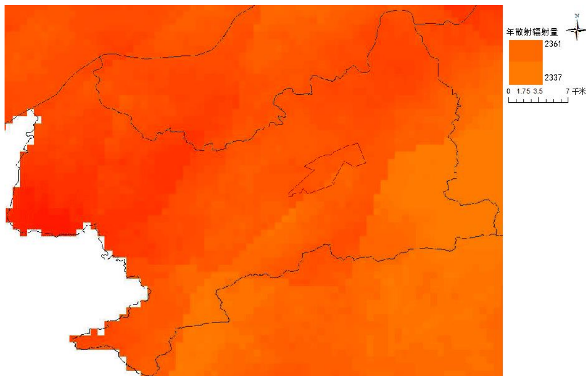
图 7.1-4 中伙现代生态产业园太阳年散射辐射量空间分布
