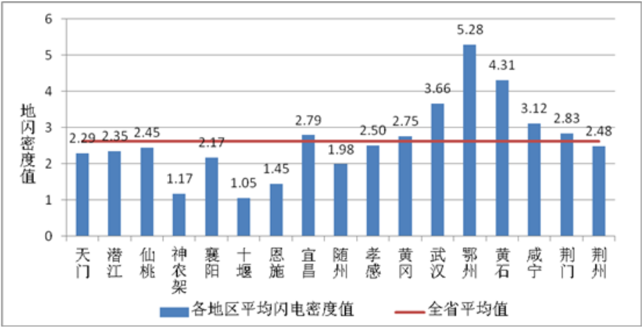
图6.3-4 湖北省2007-2018年平均地闪密度区域分布（单位为次 \text{km}^{-2} \text{ a}^{-1} ）
