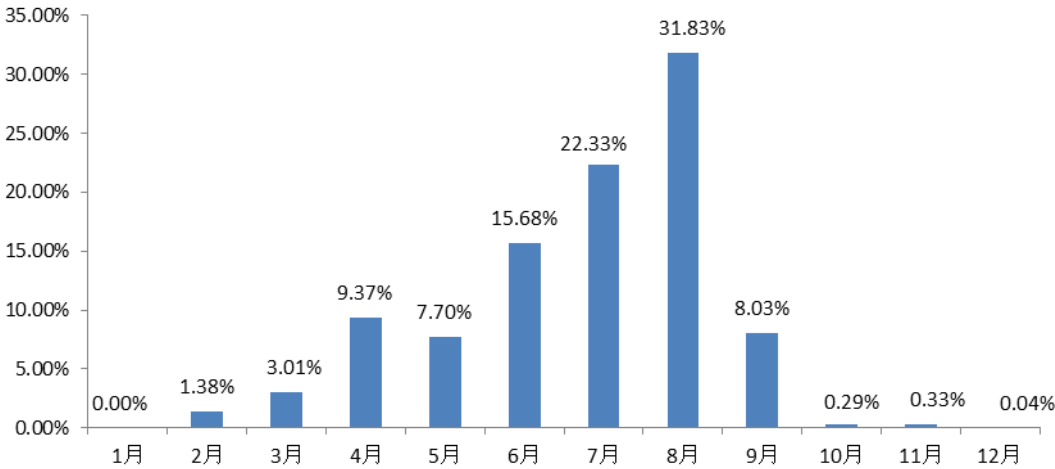
图 5.2-4 2007-2018 年赤壁中伙现代生态产业园及周边地闪回击月变化特征
