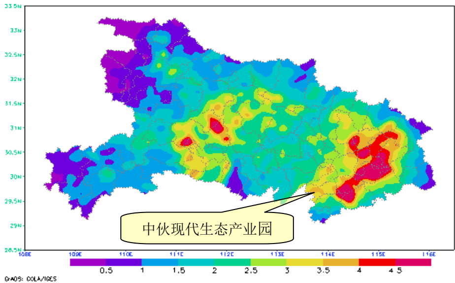
图 6.3-3 2007-2018 年湖北省平均地闪密度分布（单位为次·km 2 ·a -1 ）
