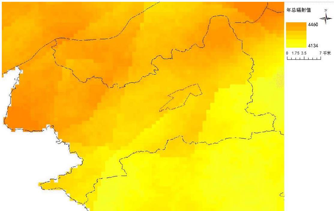
图 7.1-2 中伙现代生态产业园太阳年总辐射量空间分布
