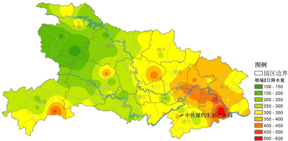
图 5.1-10 1961-2018 年湖北省极端 2 日降水量分布图
