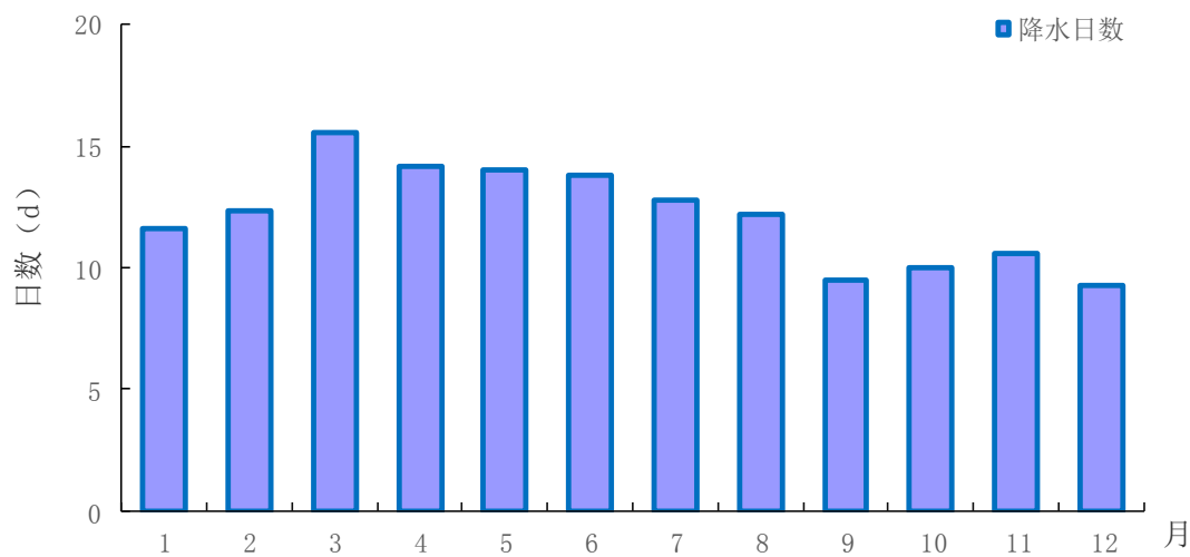
图 4.3-4 赤壁气象站累年（1989-2018 年）降水日数年变化
