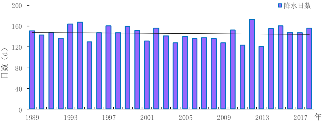
图 4.3-3 赤壁气象站 1989-2018 年降水日数年际变化
