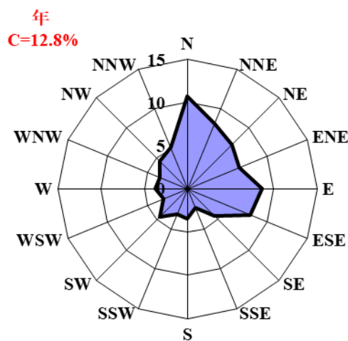
图 4.4-8 赤壁气象站累年（1989-2018 年）四季及年风向频率（%） 2016-2018 年资料完整时段，赤壁气象站、中伙铺、莲花塘区域站四季和年各风向频率（表 4.4-7、4.4-8、4.4-9）。
