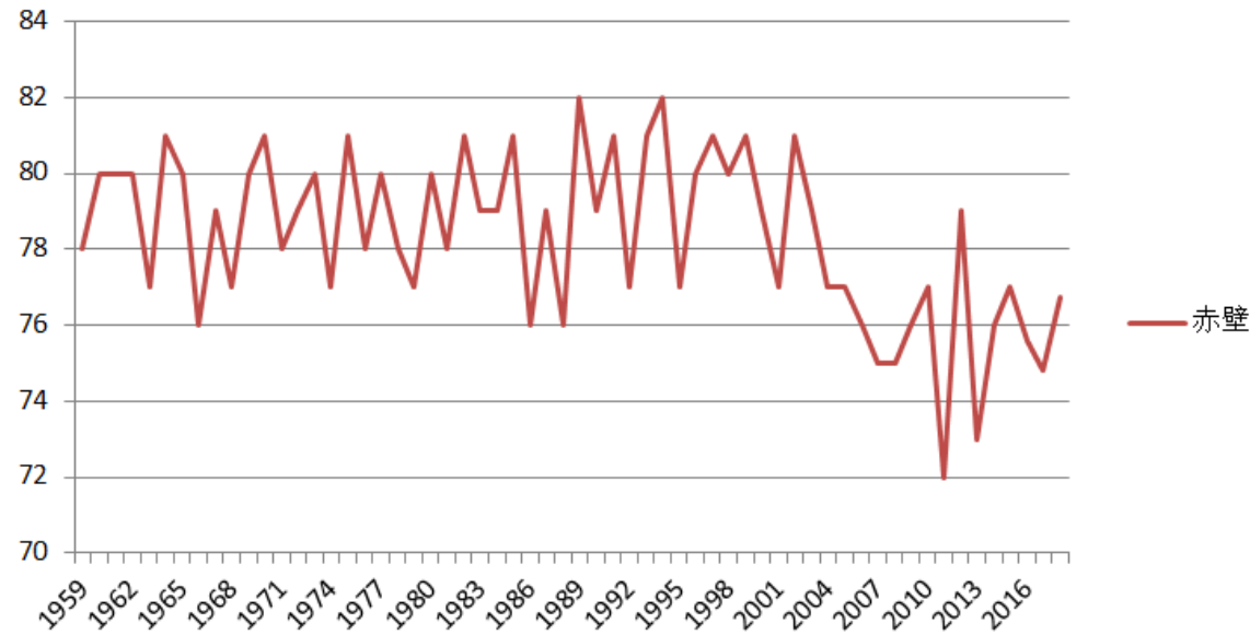
图 3.2-3 (c) 建站至 2018 年平均相对湿度年际变化
