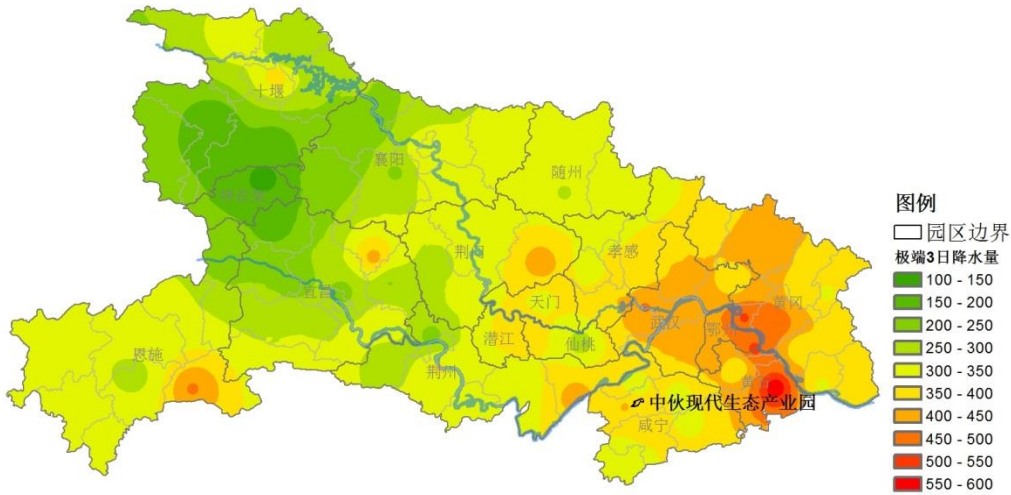
图 5.1-11 1961-2018 年湖北省极端最大 3 日降水量分布图
