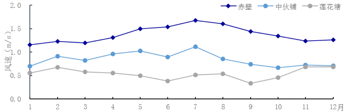
图 4.4-5 赤壁气象站和中伙铺、莲花塘区域站（2016-2018 年）平均风速年变化
