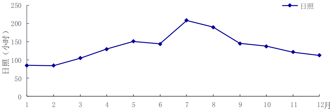
图 4.6-2 赤壁气象站累年（1989-2018 年）日照年变化
