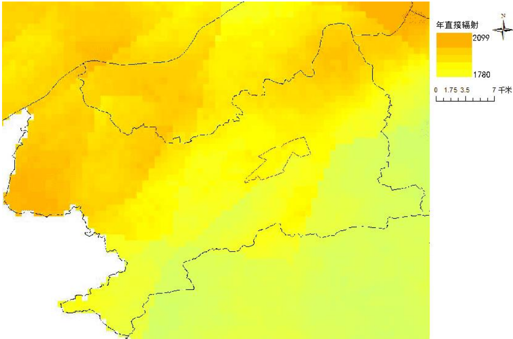
图 7.1-3 中伙现代生态产业园太阳年直接辐射量空间分布
