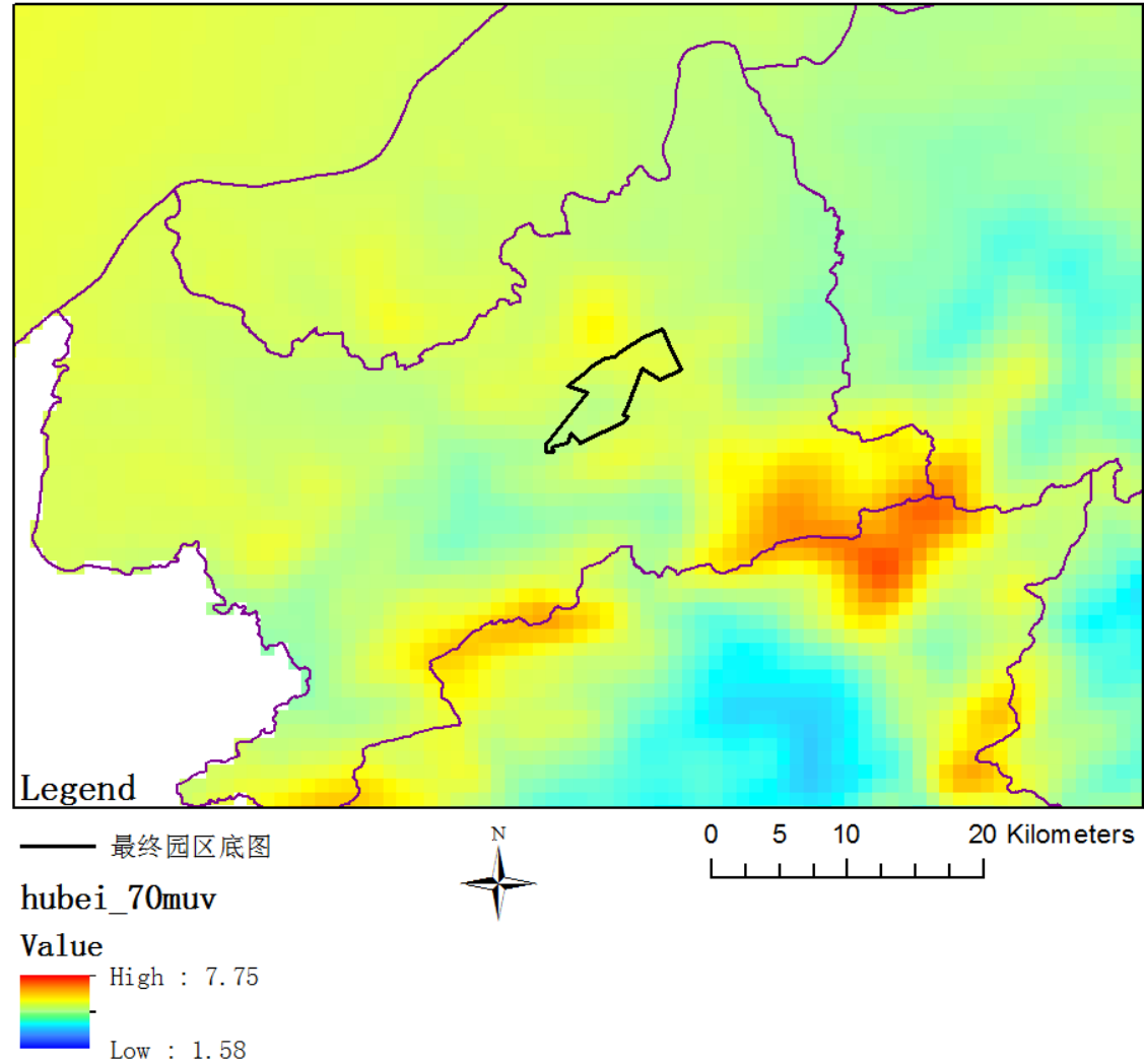
图 7.2-1 中伙现代生态产业园风速空间分布模拟
