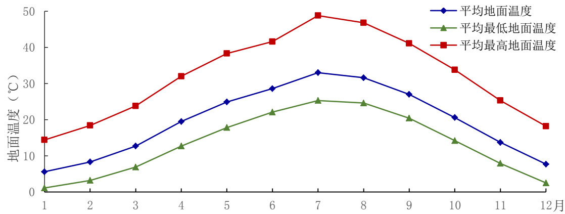
图 4.7-4 赤壁气象站累年(1989-2018 年)
