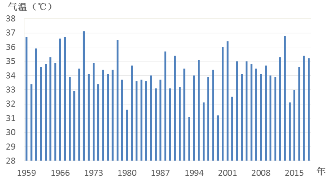
图 5.5-1 赤壁气象站最高温度月的月平均最高气温年际变化图（1959-2018 年）
