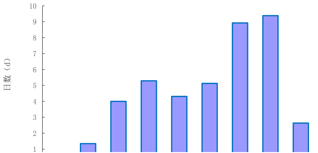
图6.2-2 赤壁气象站累年（1959-2013年）雷暴平均日数年变化
