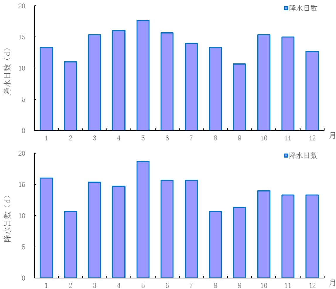
图 4.3-5 赤壁气象站、中伙铺、莲花塘区域站（2016-2018 年）降水日数年变化
