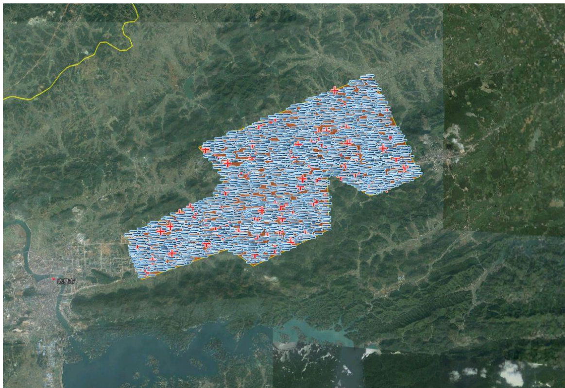
图 5.2-1 2007-2018 年赤壁中伙现代生态产业园及周边地闪回击示意图
