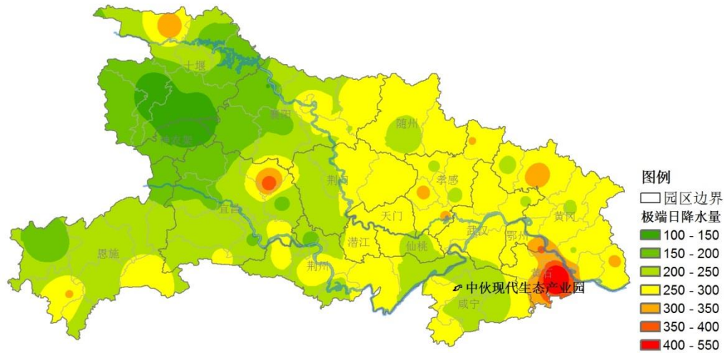
图 5.1-9 1961-2018 年湖北省极端最大日降水量分布图
