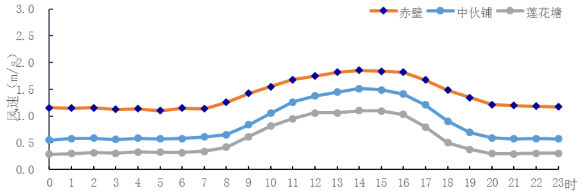
图 4.4-7 赤壁气象站和中伙铺、莲花塘区域站（2016-2018 年）平均风速日变化
