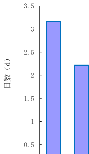
图 6.5-2 赤壁气象站 1959-2018 年积雪平均日数年变化
