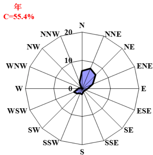
图 4.4-7 赤壁气象站、中伙铺、莲花塘区域站（2016-2018 年）四季及年风向频率（%）
