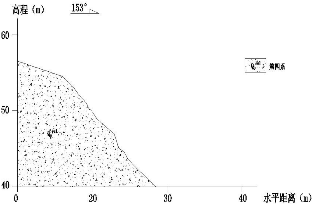
图4-1 (QP11) 切坡高程剖面示意图
