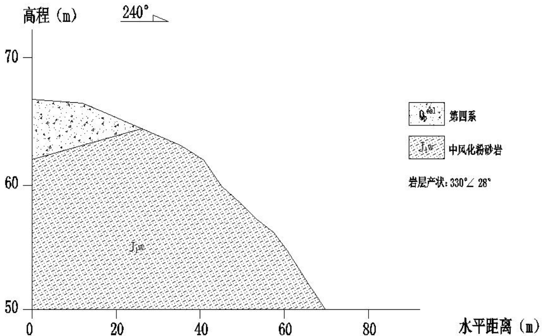
图4-2 (QP7) 切坡高程剖面示意图
