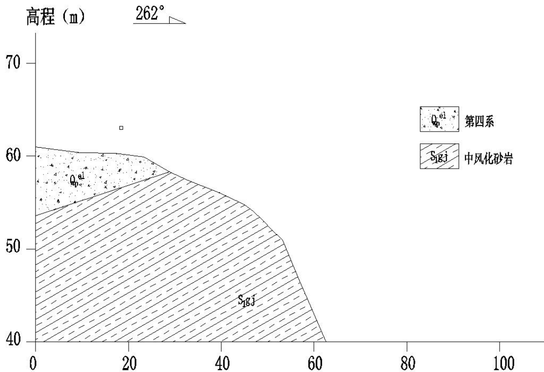
图4-2 (QP3) 切坡高程剖面示意图
