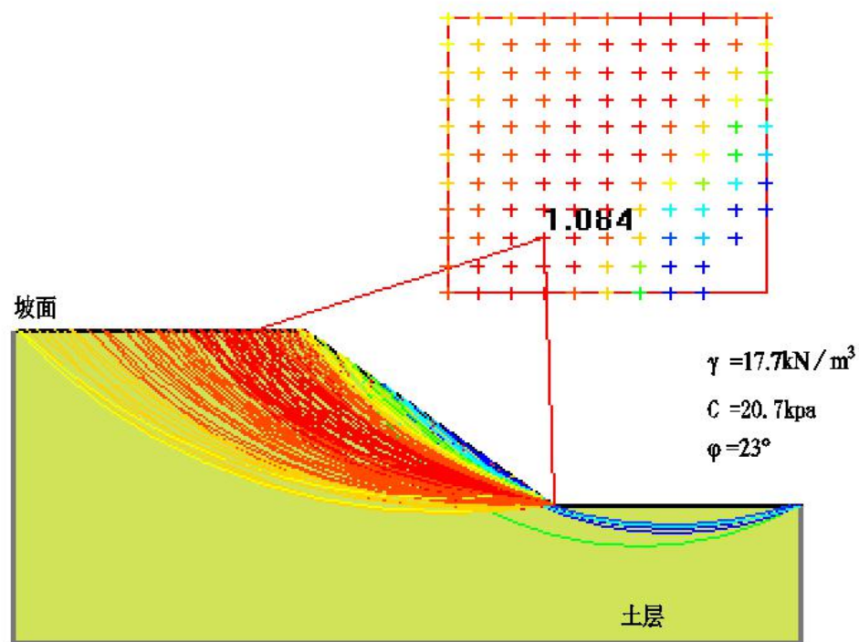
图4-2 土体正常工况条件下边坡稳定系数计算过程
